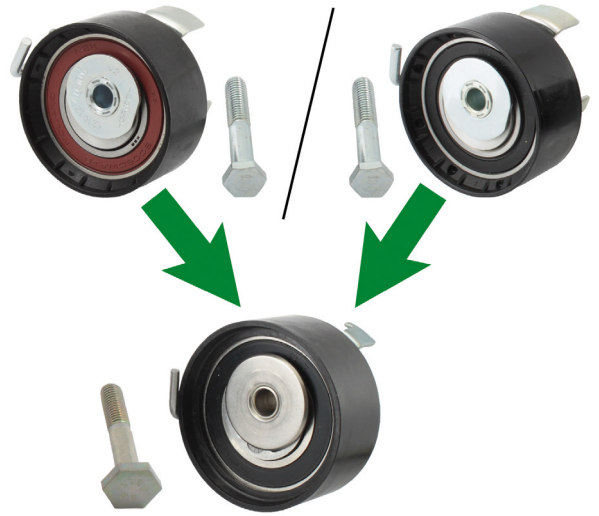
Kuva 1: Ylempänä näkyy tähänastinen malli punaisella tai mustalla tiivisteellä/alempana on uusi malli
