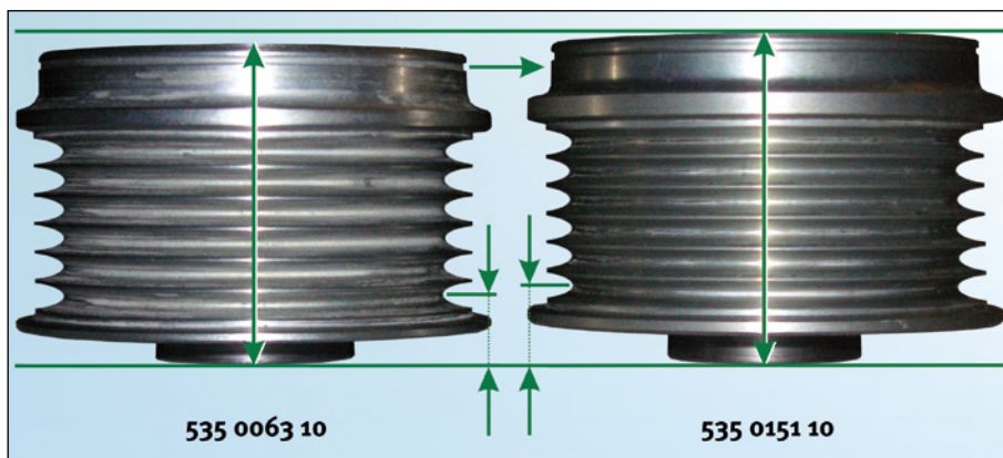
Fig 3: Diferenciación entre la polea libre del alternador INA 535 0063 10 (VALEO) y 535 0151 10 (DENSO)
