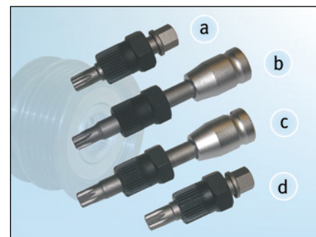
Fig 2: Vista general de las herramientas especiales
